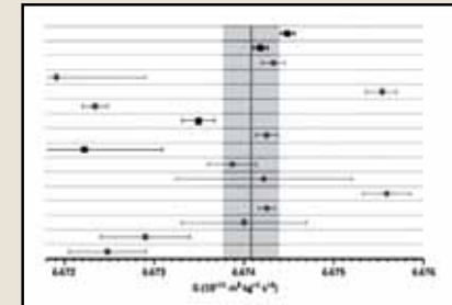
萬有引力G值。
