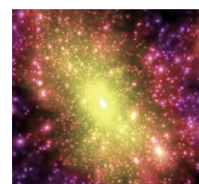
關於暗物質的電腦模擬圖(網路照片)
