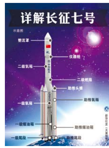
詳解長征七號。(新華社 大巢製圖)
